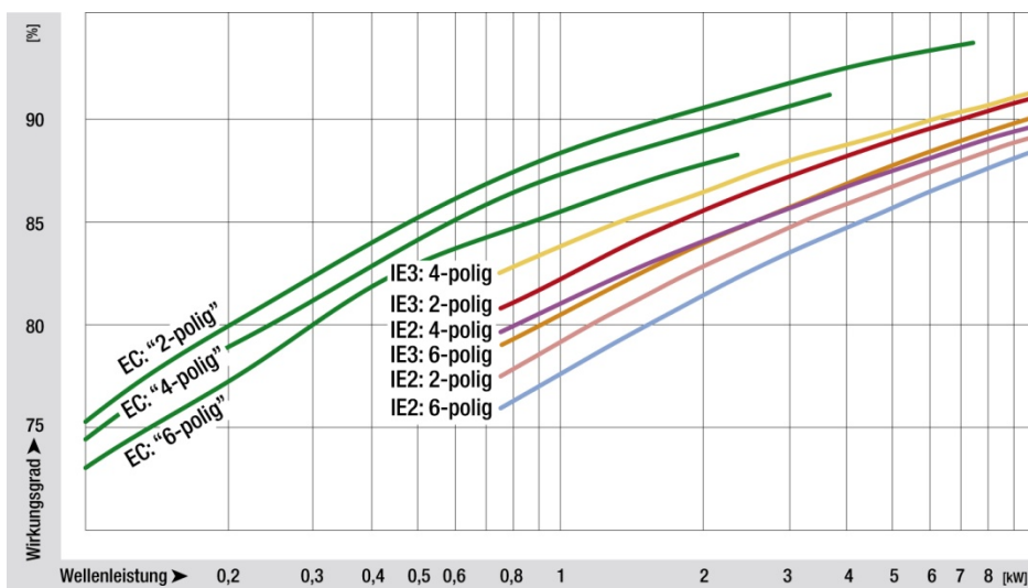
Obrázek 2: porovnání EC a AC motorů s požadovanými křivkami účinnosti
